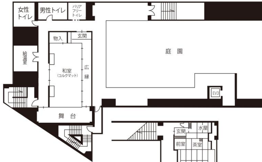
5階平面図 使用しない
